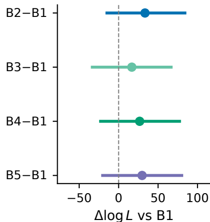
FineWeb 24B
